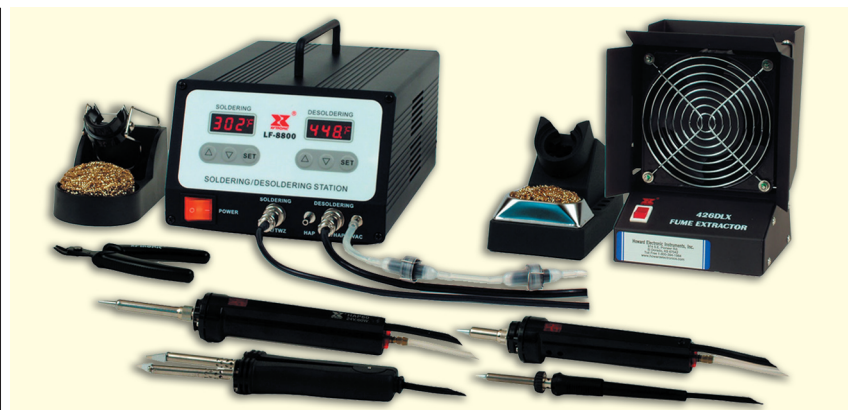
Рис. 3. Микропроцессорная цифровая ремонтная паяльная станция LF-8800TP
